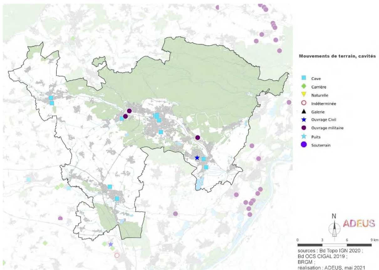
Carte n°41. Localisation des zones de mouvements de terrain, cavités
