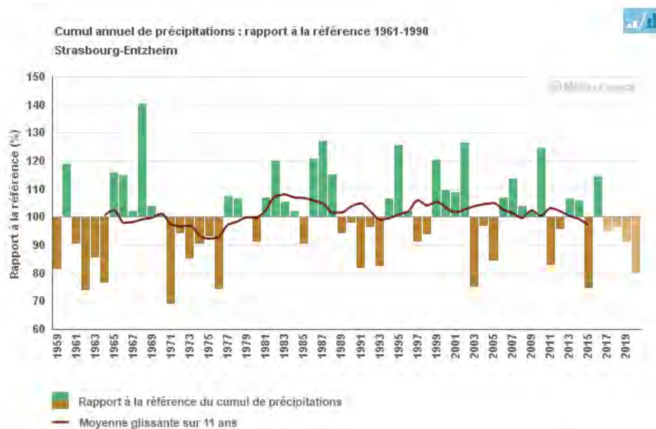
Graphique n°10. Cumul annuel de précipitations
