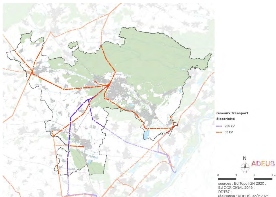
Carte n°57. Réseau de transport d'électricité
