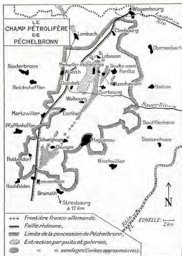
Fig. 1 - Le champ pétrolifère de Pechelbronn.
